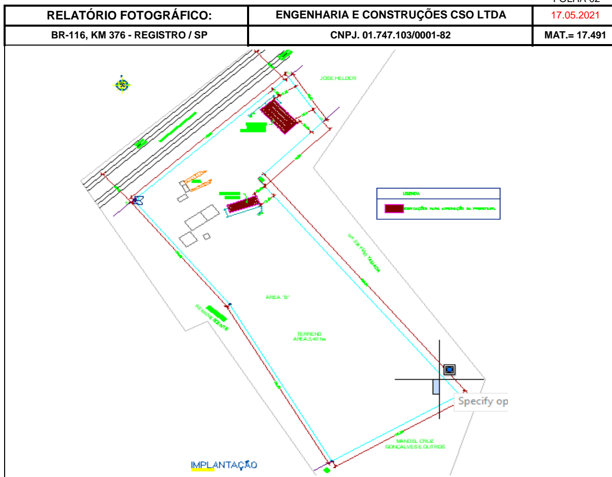
FOTO 03= PLANTA DE LEVANTAMENTO TOPOGRÁFICO DA ÁREA DO IMÓVEL
